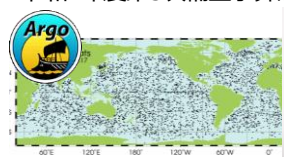
アルゴ計画/アルゴフロート
