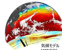
独自の全球気候モデル
